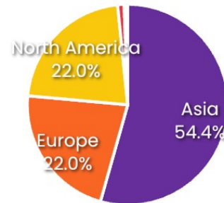
IETF Meeting 122
