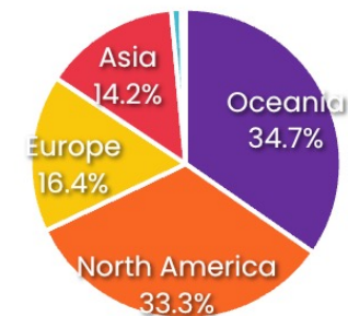
IETF Meeting 119
