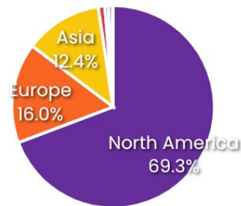
IETF Meeting 120
