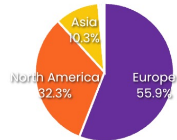
IETF Meeting 121
